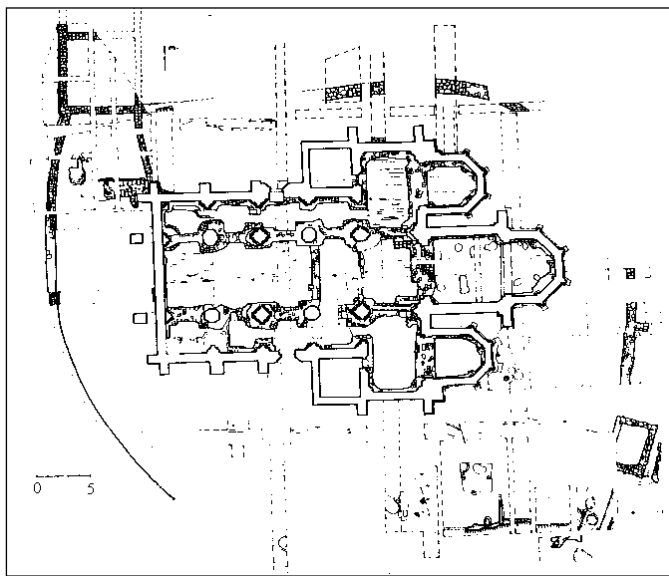
4. ábra: A régészeti feltárást összesítő rajza (Lukács-Cabello-Csengel 1991.)
